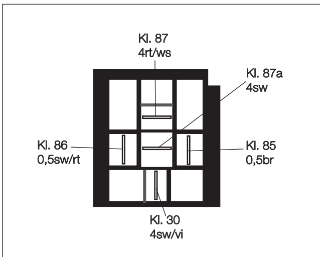
Skizze 7 Anschlüsse des Relais 2.5.7 von der Kabeleintrittsseite betrachtet
