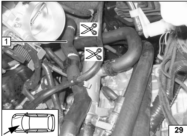
1 Schlauch Motoraustritt
