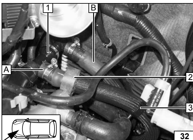
1 Rückschlagventil 2 Distanzgummi 3 Schlauchhalter
