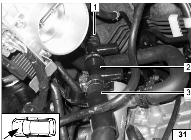
1 Schlauchstück Wärmetauschereintritt 2 Rückschlagventil 3 Schlauchstück Motoraustritt
