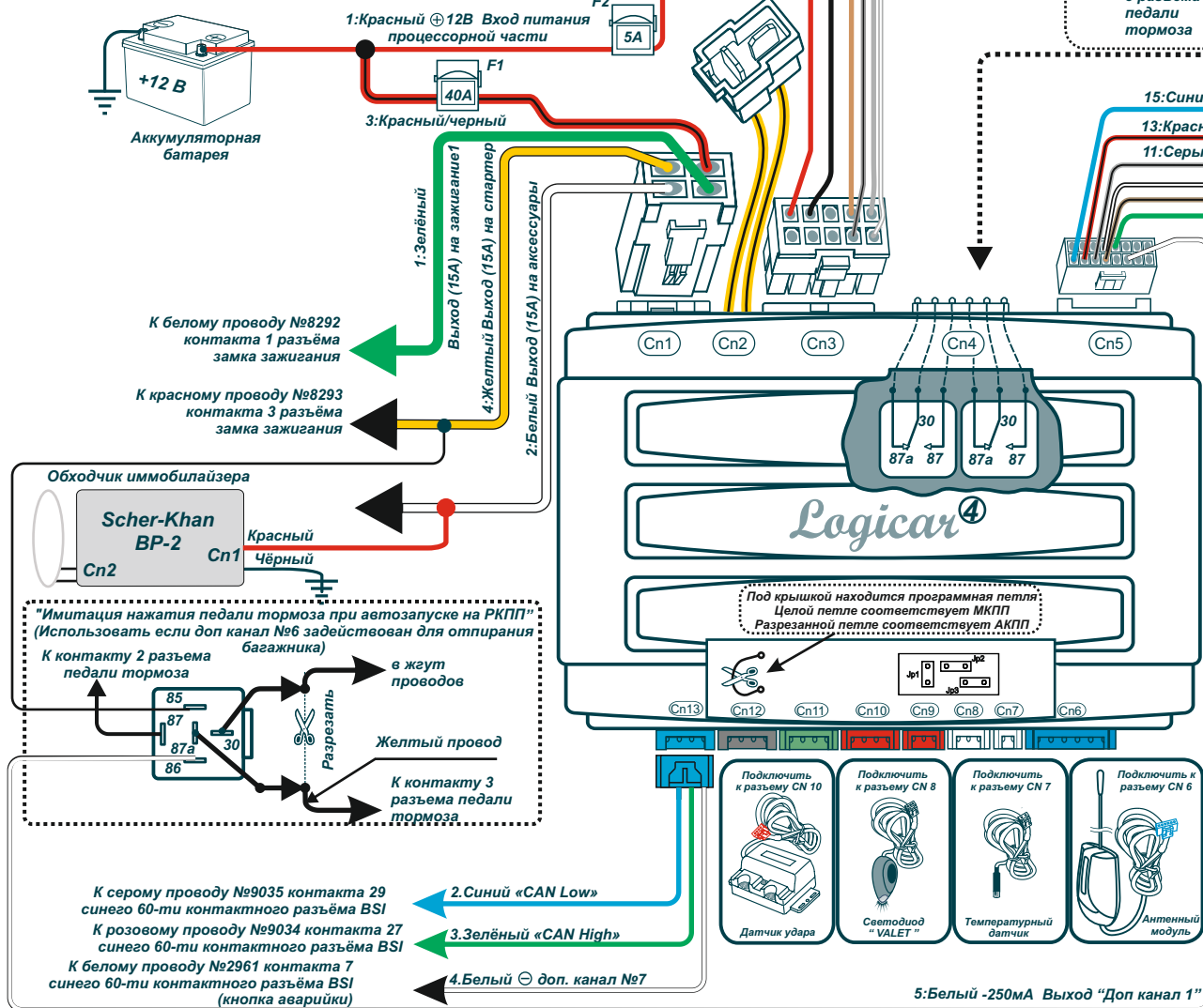
Схема подключения Scher-Khan Logicar 4 к автомобилю Citroen C-Elysee
