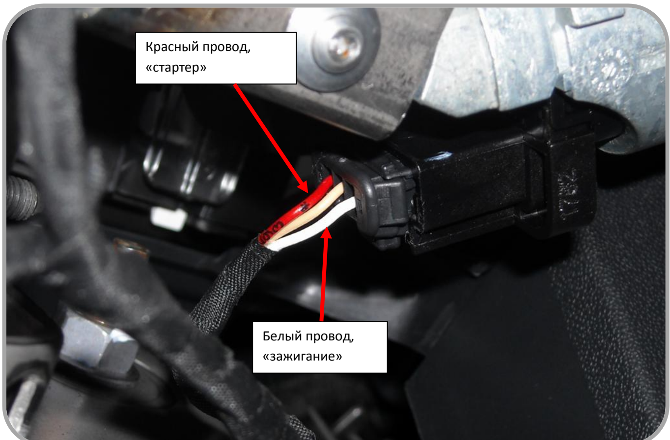
Рис. 4: Подключение цепей автозапуска.
