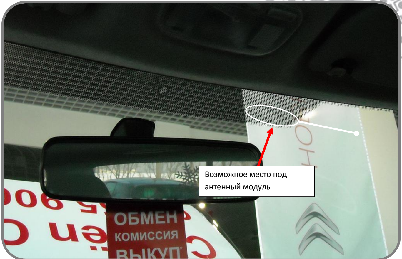
Рис. 11: Возможное место установки антенного модуля.
