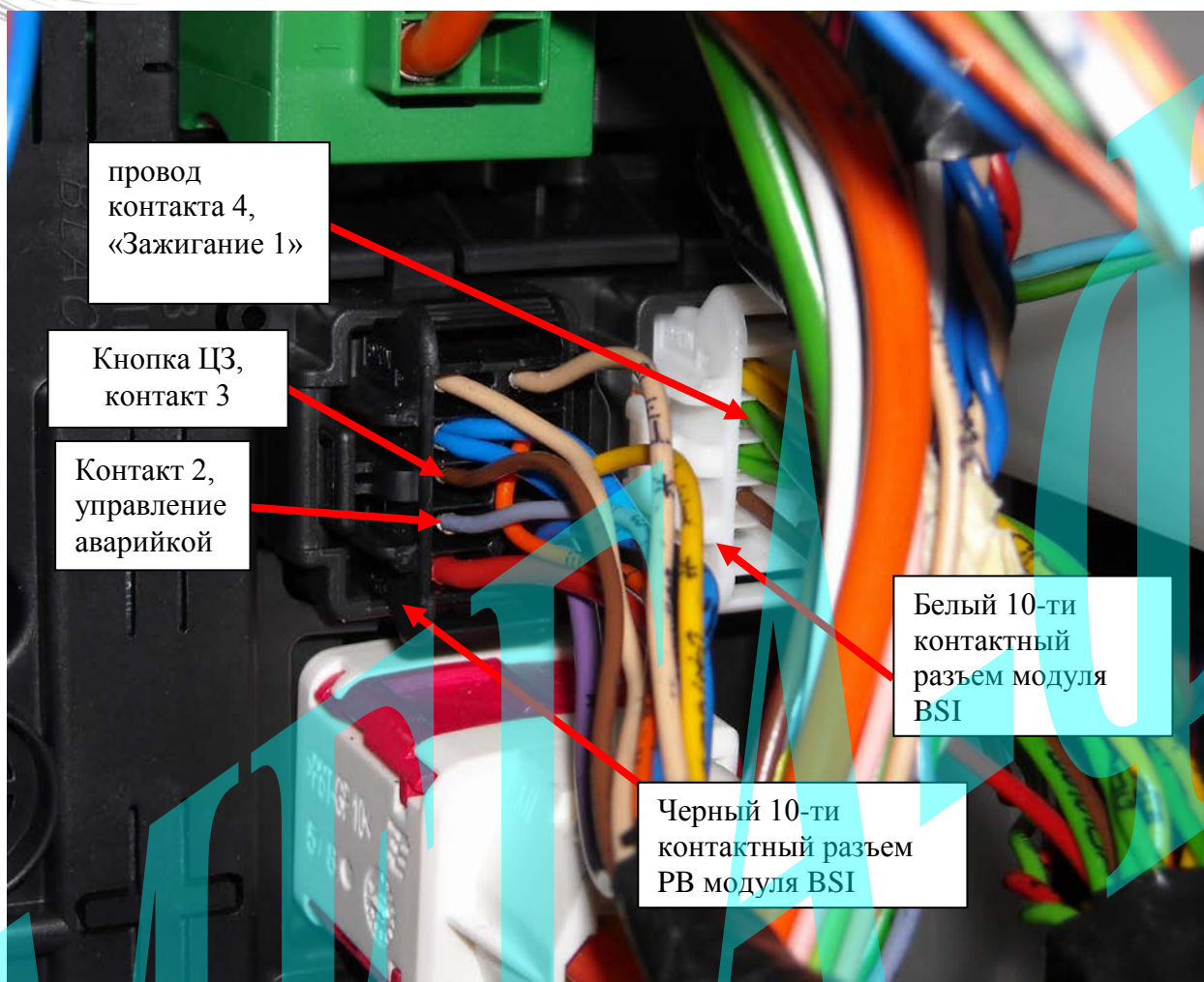
Рис. 3: Подключение к аварийке и ЦЗ.
