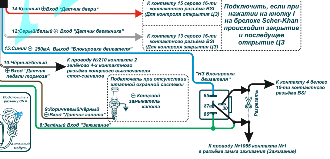
Схема подключения системы Scher-Khan Logicar 4 к автомобилю Peugeot 3008
