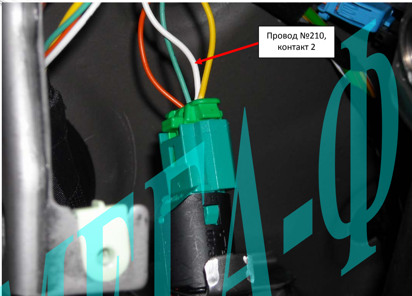
Рис. 7: Подключение датчика педали тормоза.
