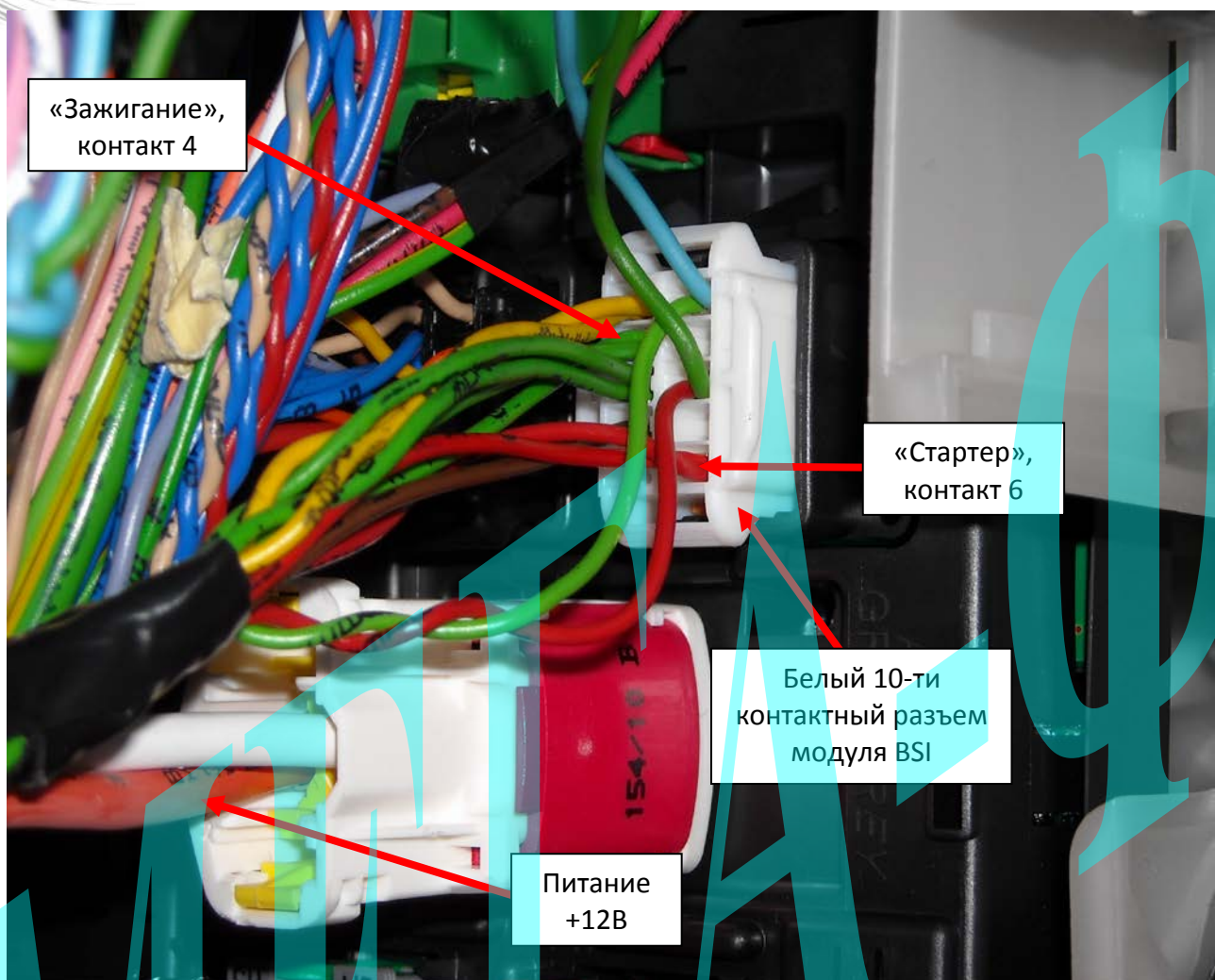
Рис. 5: Подключение цепей автоматического запуска.
