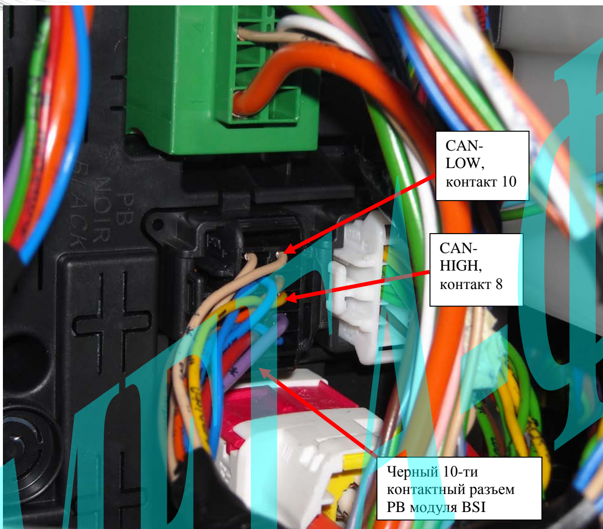
Рис. 2: Подключение к CAN шине.
