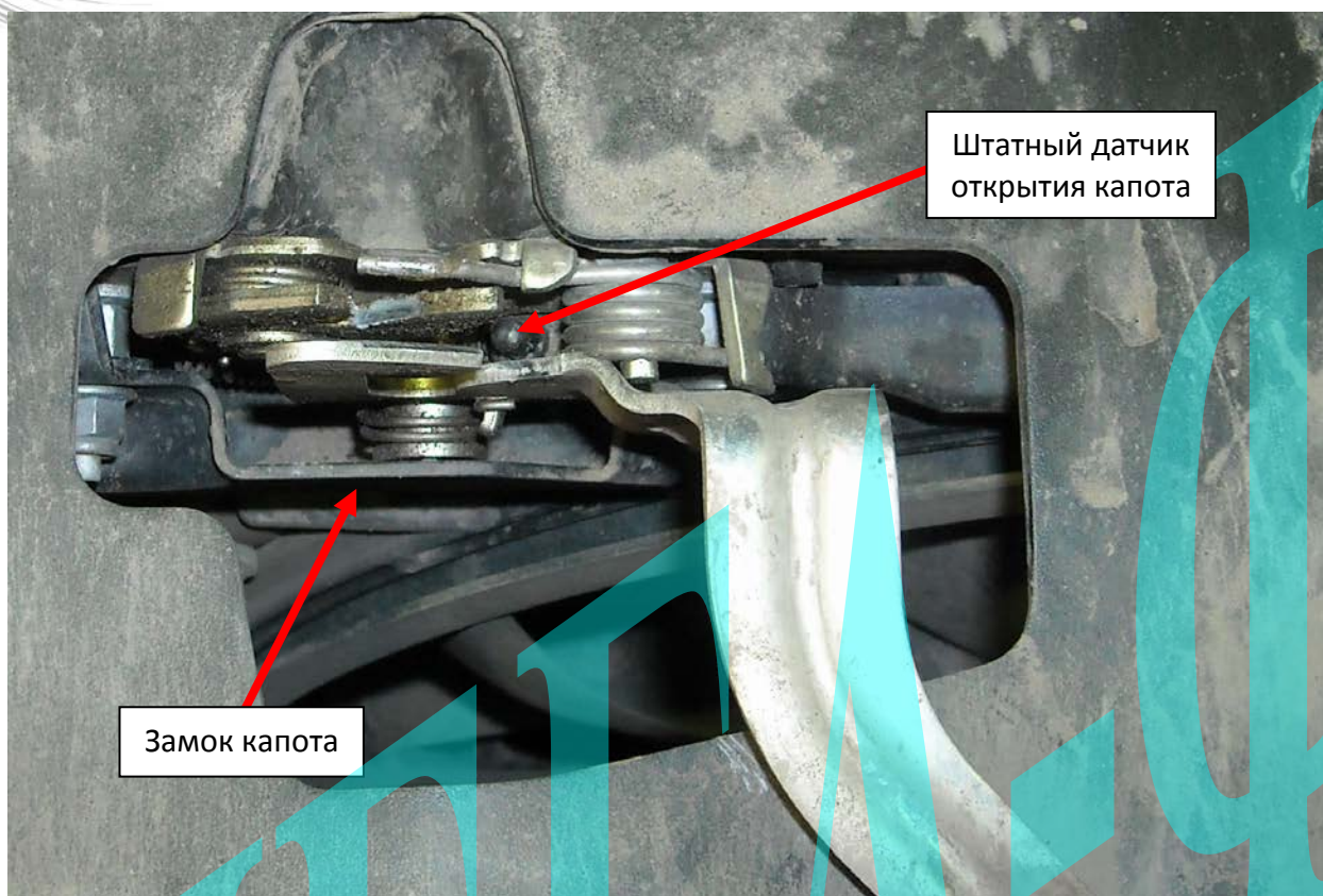
Рис. 8: Штатный концевик капота.
