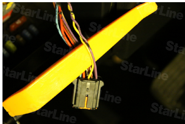
Фото 8.2. CAN-шина (Pin № 8,10)
