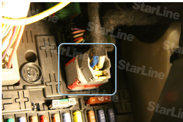
Фото 12. Постоянный плюс (синий или белый)
