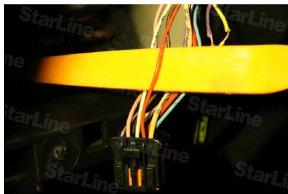
Фото 8.4. Аварийка (Pin №2)
