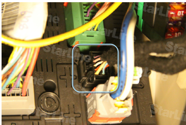
Фото 8.1. 10-контактный разъем
