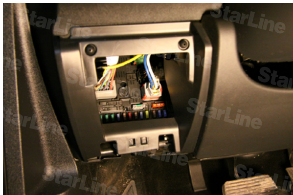
Фото 2.1. Снятие кармана
