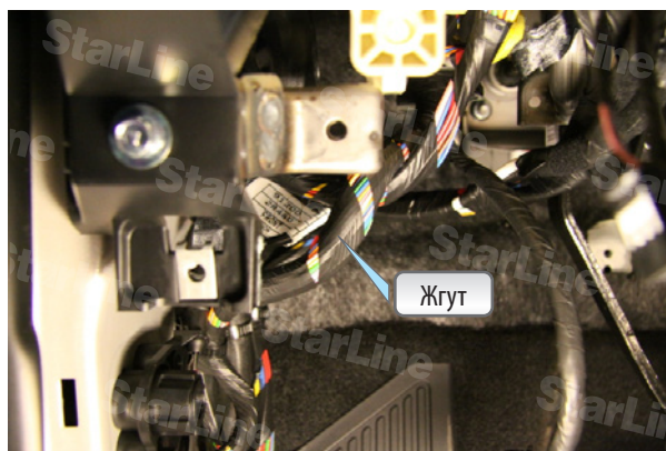
Фото 14.1. Жгут
