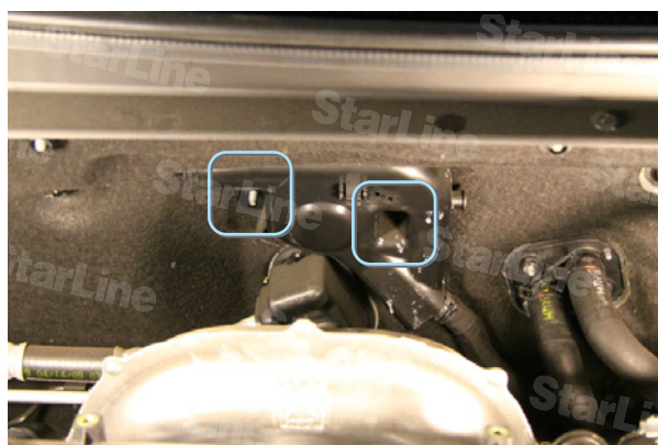
Фото 6.5. Крышка штатного уплотнения (крепление на 2 гайки М6)
