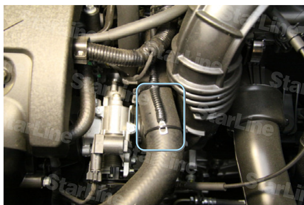
Фото 6.3. Датчик температуры
