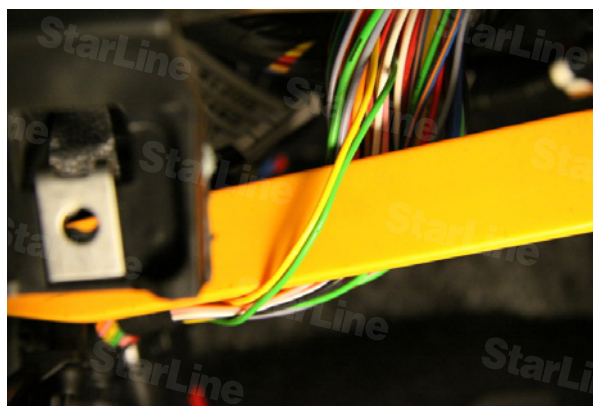
Фото 14.2. ЦЗ (зеленый и желтый)
