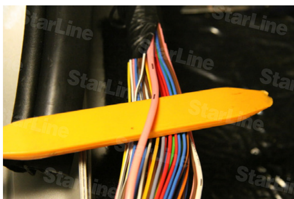
Фото 19. Бензонасос (розовый)
