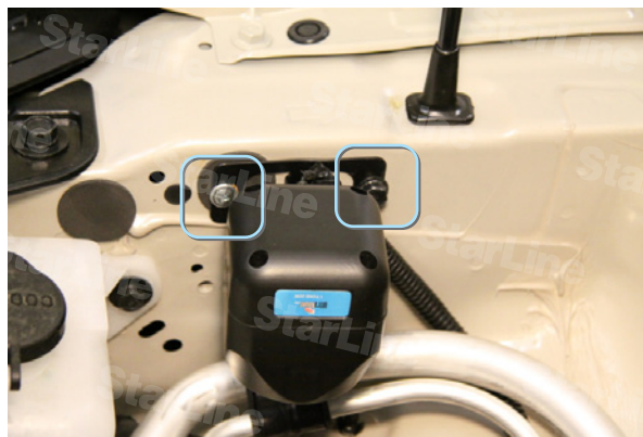
Фото 6.2. Крепление сирены
