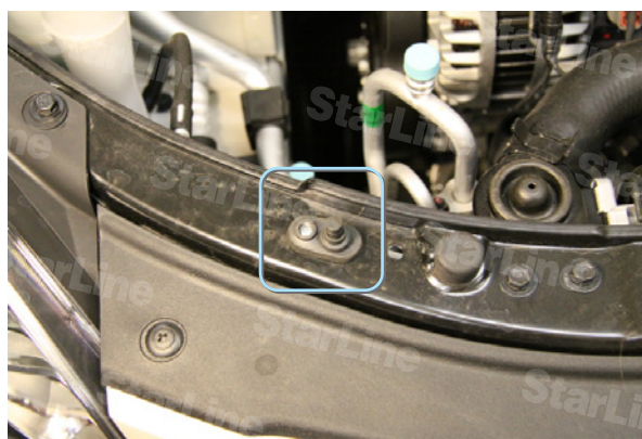
Фото 6.4. Концевик капота (отрезать 2 деления)
