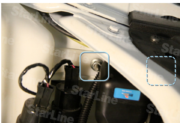
Фото 5.2. Сирена. Крепление гайкой М6 и саморезом
