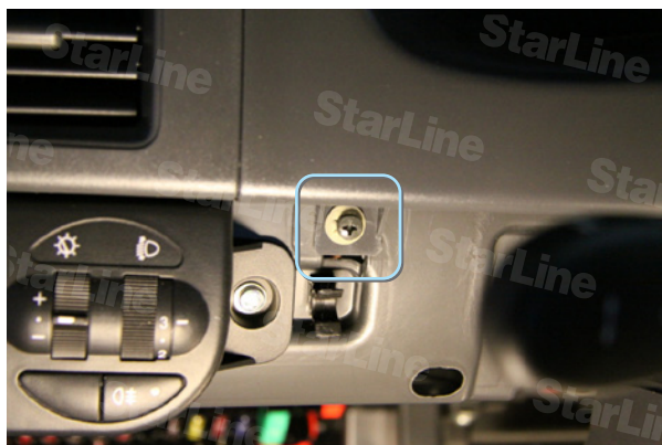
Фото 1.5. Крепление облицовки приборного щитка
