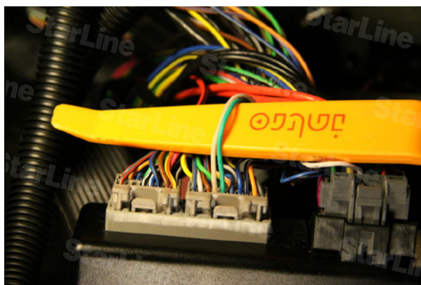
Фото 17. Провода рамки штатного иммобилайзера (белый, зеленый)
