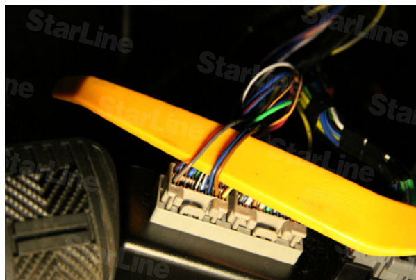
Фото 11.1. Концевики дверей (сине-черный, коричневый, серо-оранжевый)
