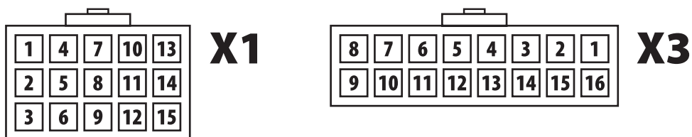
Нумерация контактов разъемов. Вид со стороны проводов
