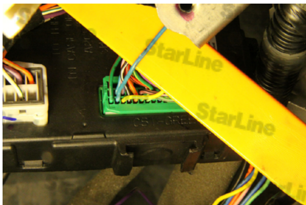
Фото 12. Концевик водительской двери (голубой)
