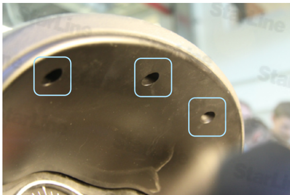
Фото 3.1. Крепление облицовки
