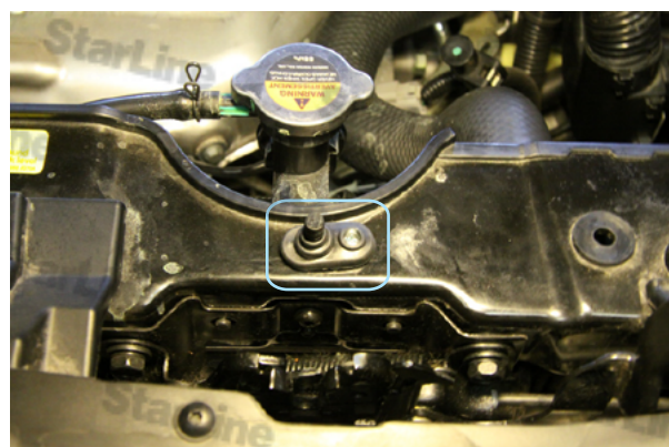
Фото 4.4. Концевик (отрезать 3 деления)
