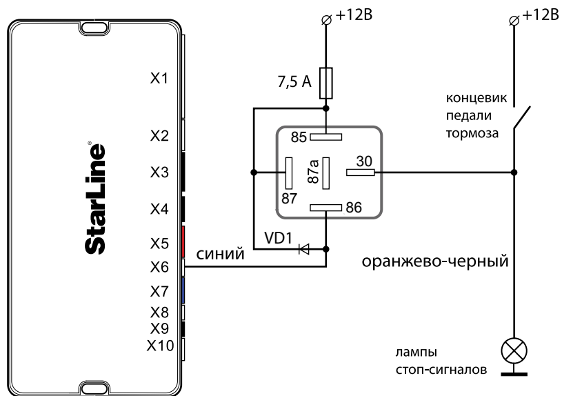
Схема 1. Имитация нажатия педали тормоза
