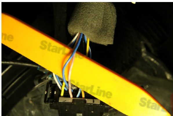
Фото 11. CAN-шина (CAN-H синий, CAN-L розовый)
