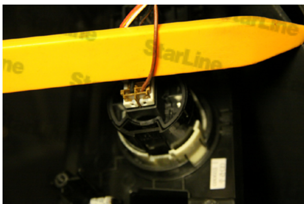
Фото 10. Старт-Стоп (коричневый)
