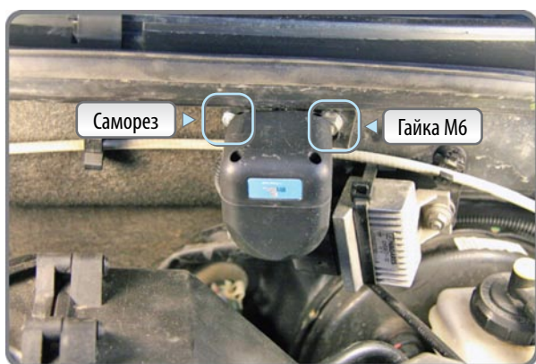
Фото 6.1. Крепление сирены
