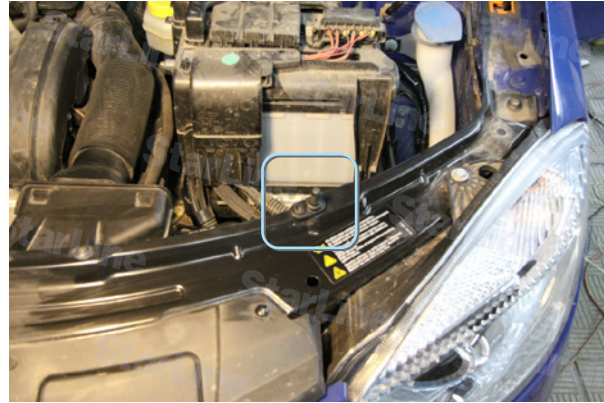
Фото 4.4. Концевик капота
