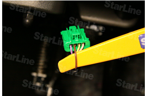
Фото 13.2. Тормоз (коричневый pin №2)
