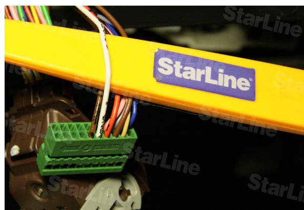
Фото 11.2. Центральный замок (белый pin15)
