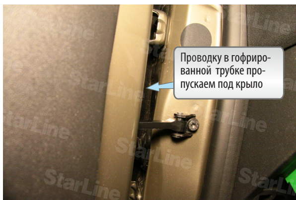
Фото 4.3. Прокладка жгута в подкапотное пространство через крыло
