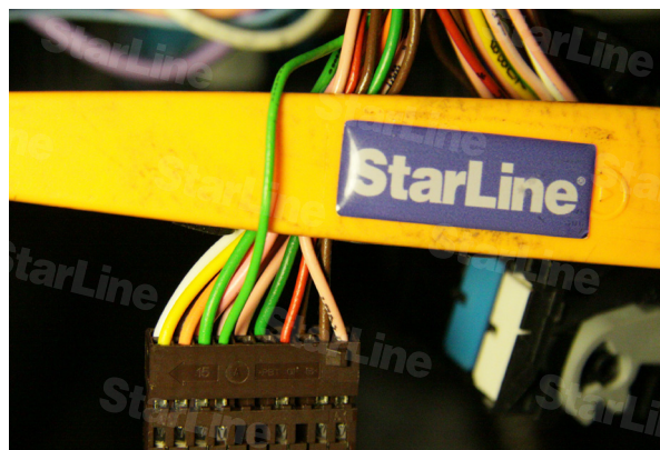
Фото 10.2. Передний левый указатель поворотов (зеленый pin57)
