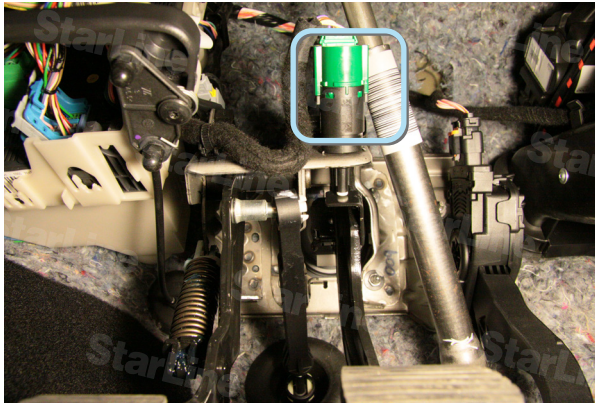
Фото 13.1. Расположение разъема концевика педали тормоза
