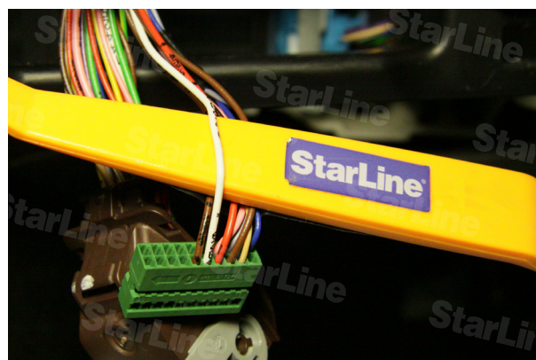
Фото 9.2. Концевик водительской двери (белый pin15)
