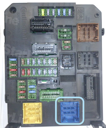
Фото 15.1. Разъем FPB Bleu (синий) в блоке BSI
