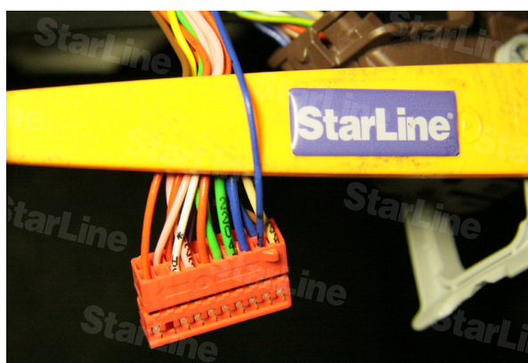
Фото 10.6. Задний правый указатель поворотов (синий pin52)
