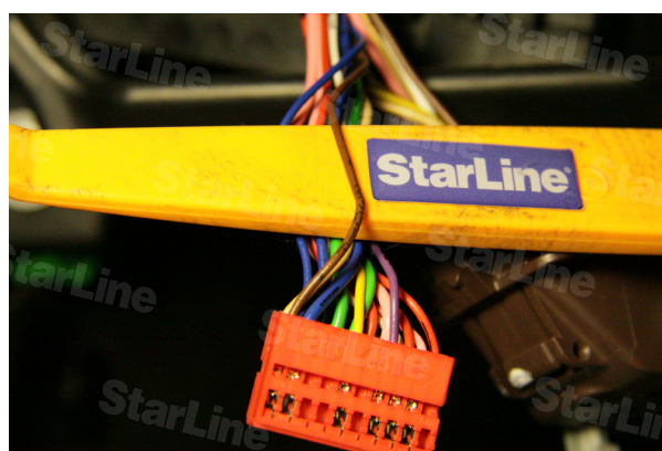
Фото 10.5. Задний левый указатель поворотов (коричневый pin41)
