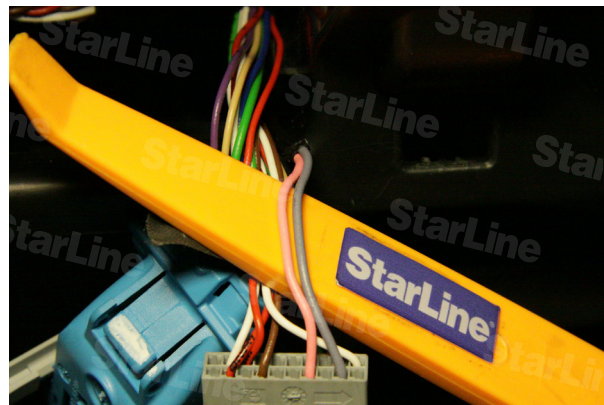
Фото 8.2. CAN-H (розовый pin27), CAN-L (серый pin29)
