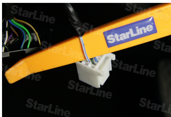
Фото 8.2. Ручной тормоз (бело-синий 8pin)
