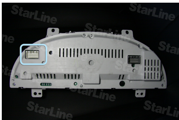
Фото 10.1. Местоположение разьема
