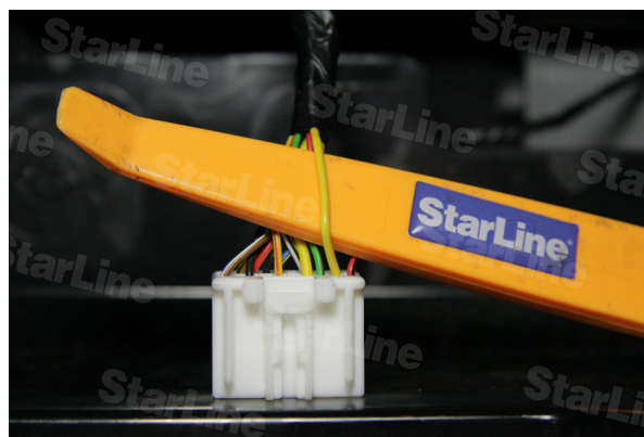
Фото 10.2. Провод контрольной лампы зарядки (желтый)
