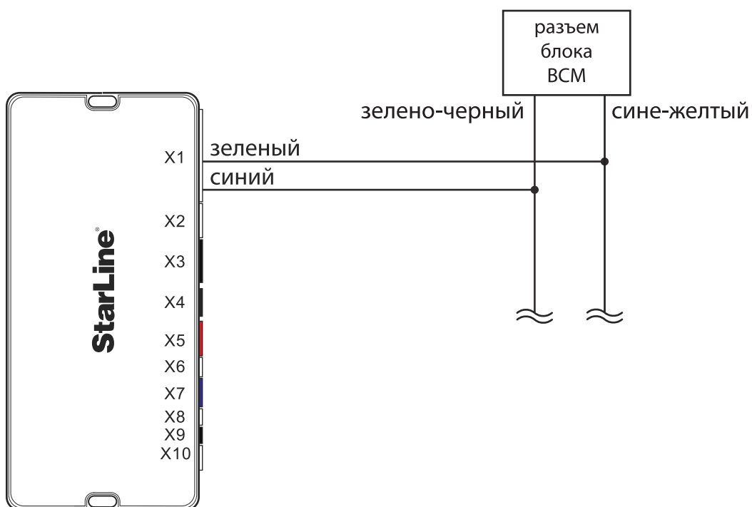
Схема 2. Подключение центрального замка
