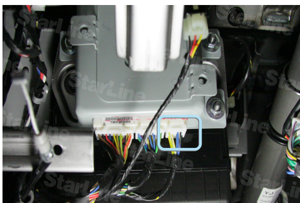
Фото 8.1. Метоположение разъема
