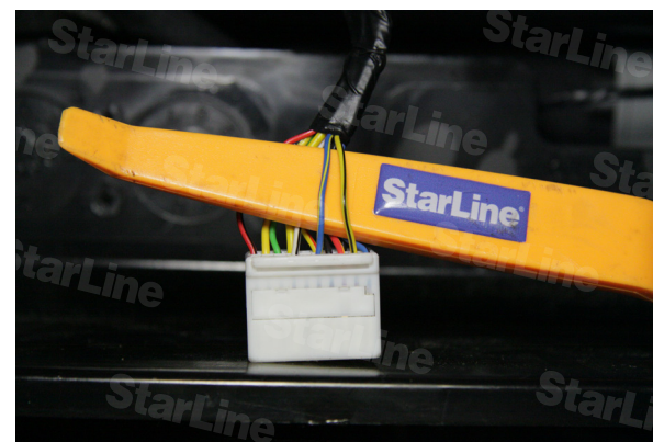
Фото 13.2. Указатели поворотов (сине-желтый, желто-черный)
