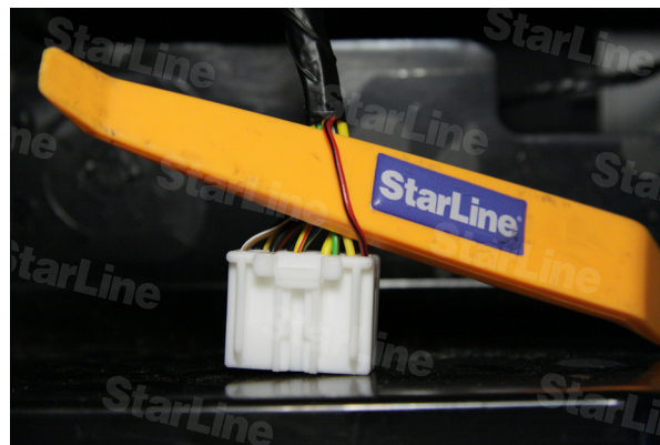
Фото 12.2 Концевики дверей и багажника (красно-черный)
