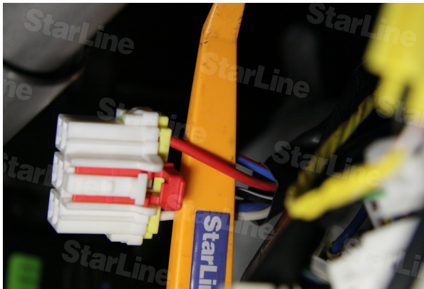
Фото 16.3. Зажигание 2(красный)
