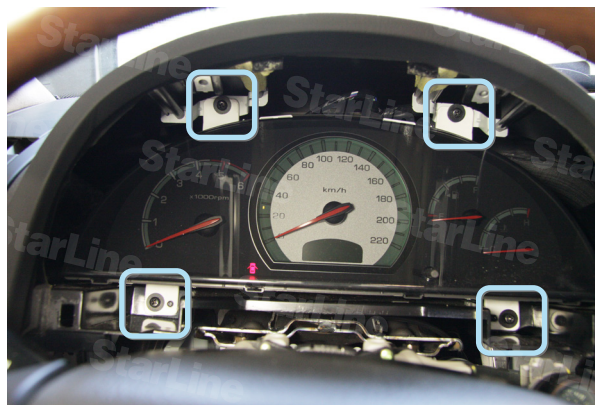
Фото 3.2. Саморезы крепления панели приборов
