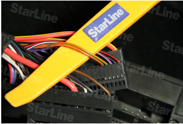
Фото 9.3. CAN-шина (CAN-H оранжево-зеленый 16pin, CAN-L оранжево-коричневый 17 pin)
