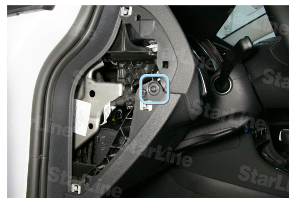
Фото 1.6. Боковое крепление подторпедника
