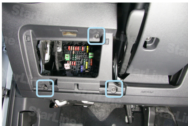
Фото 1.7. Саморезы крепления подторпедника
