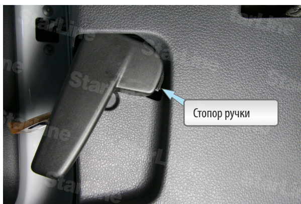
Фото 3.1. Снятие ручки открывания капота
