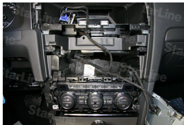
Фото 4.4. Магнитола снята
