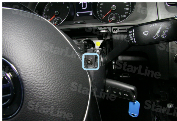
Фото 2.4. Правый саморез крепления рулевого кожуха
