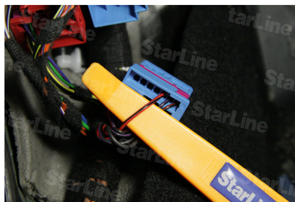
Фото 11.2. Стартер (красно-черный 5pin)
